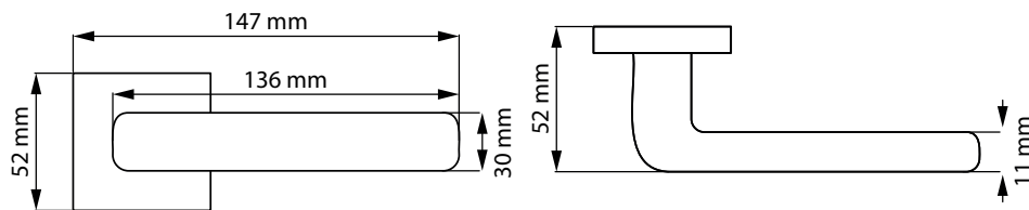
9164 MP24 CYLINDER ROSETTE Чёрный
