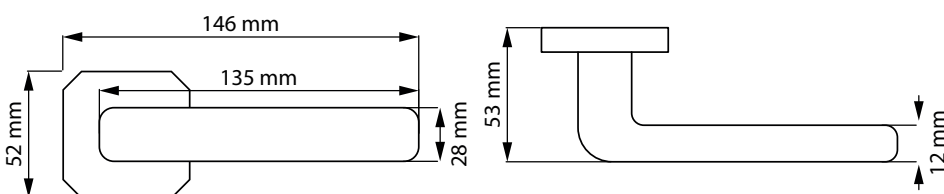
9161 MP14 CYLINDER ROSETTE Старое серебро
