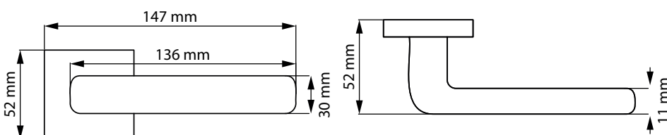
9164 MP30 CYLINDER ROSETTE Состаренная латунь
